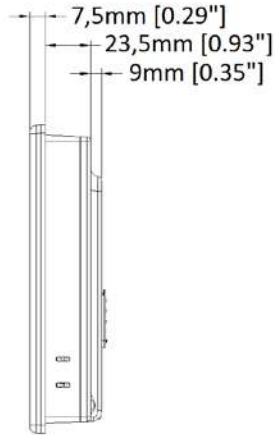
Vista Lateral
