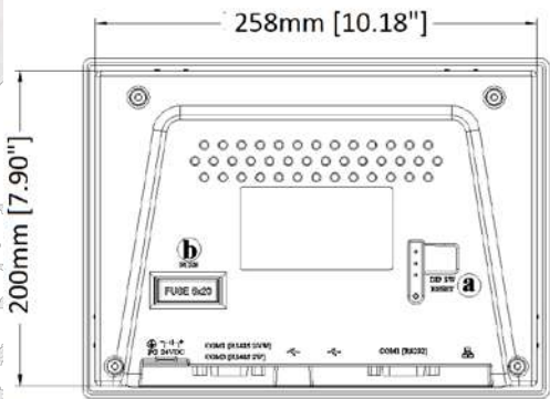
Vista Posterior
